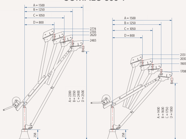
COMALU 500 T
