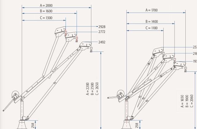
COMALU 300 T
